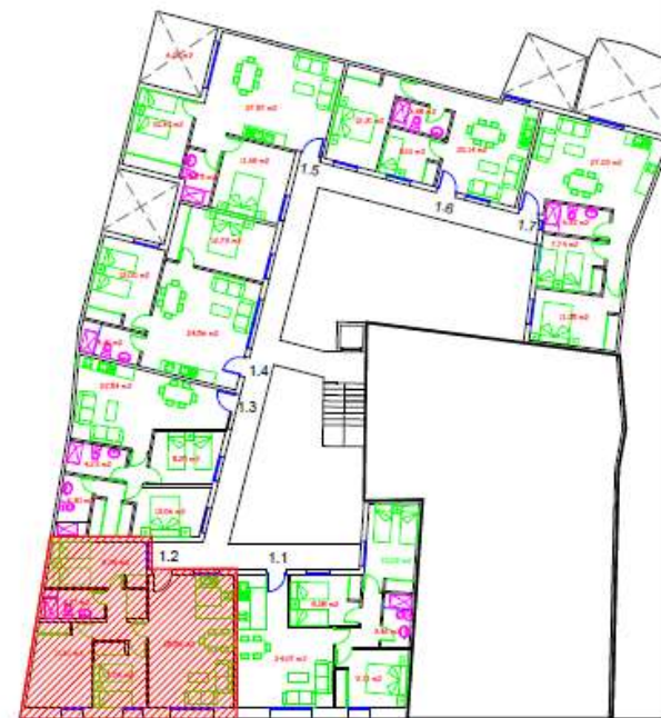
PLANTA PRIMERA CARMEN VIEJO 51
