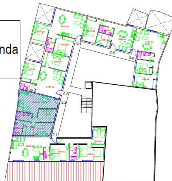
PLANTA SEGUNDA CARMEN VIEJO 51
