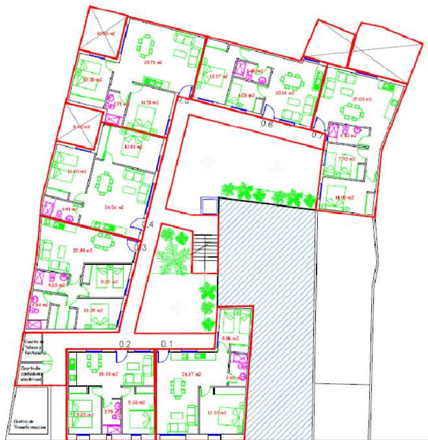
PLANTA BAJA CARMEN VIEJO 51
